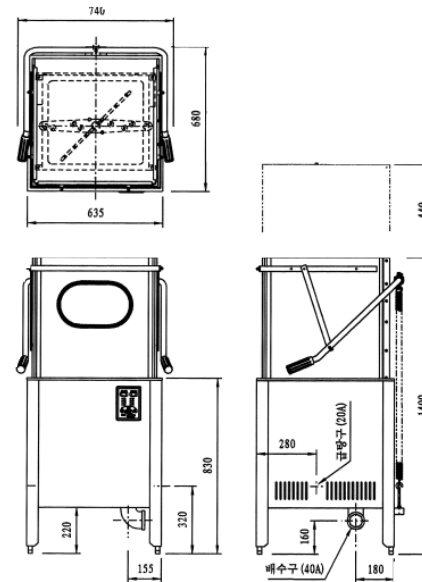
300DS 저탕식 가스부스타 Type
