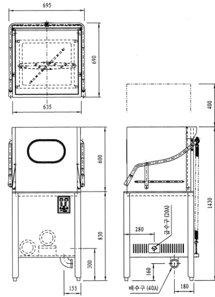
200DS 저탕식 가스부스타 Type
